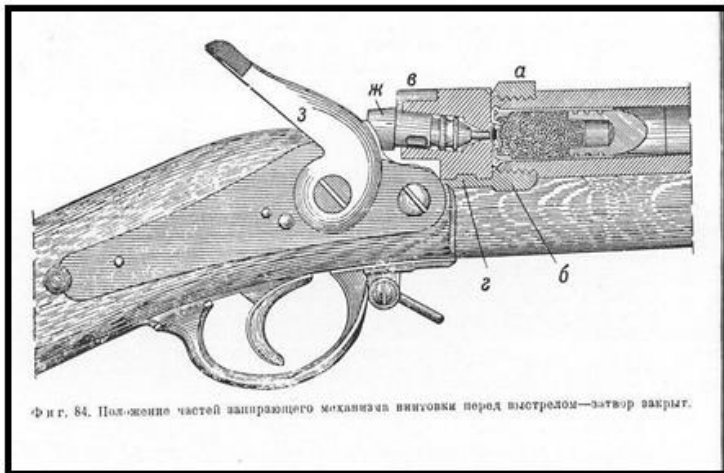
Fusil de parapeto ruso, Krnka M1876
